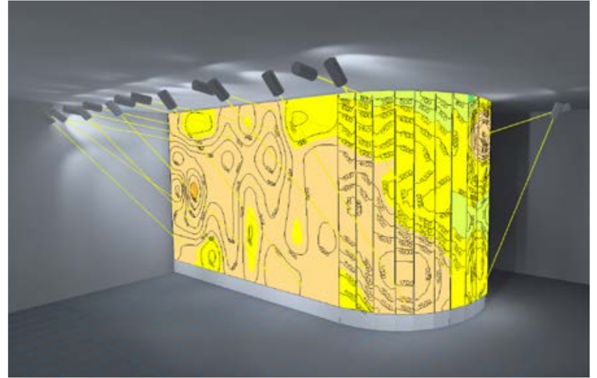
Simulation der Lichtverteilung
