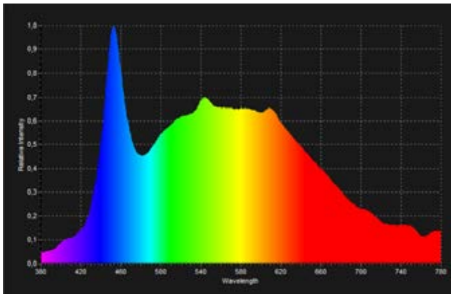
Lichtspektrum RVG-LED Chip
